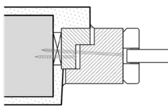
Montageleiste verputzt
