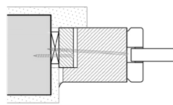
Blindstock Alu eingeputzt
