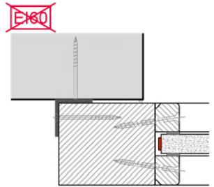
Metallwinkel verdeckt
