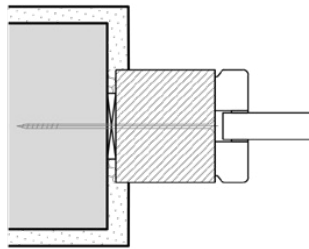
Deckleisten bündig
