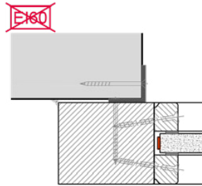
Metallwinkel in Leibung
