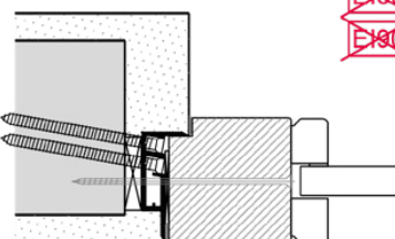
Blindstock Alu eingeputzt
