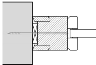
Deckleisten bündig
