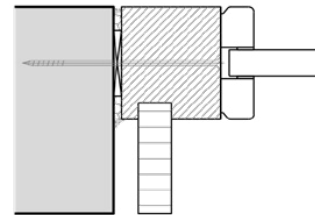
Paneelanschluss einseitig
