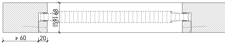
Füllung mittig Glasleisten gerade
