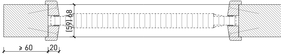
Füllung mittig, Glasleisten schräg
