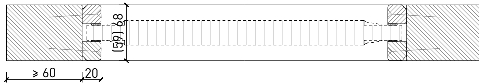
Füllung mittig Glasleisten gerade
