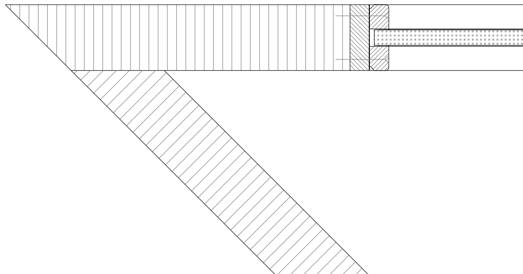
Einbau in FeuerschutzTeam Verglasung in Vollwand
